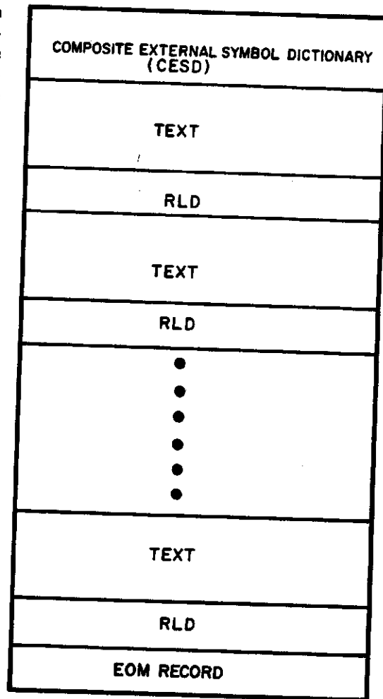
FIG. 6. Load Module format.
