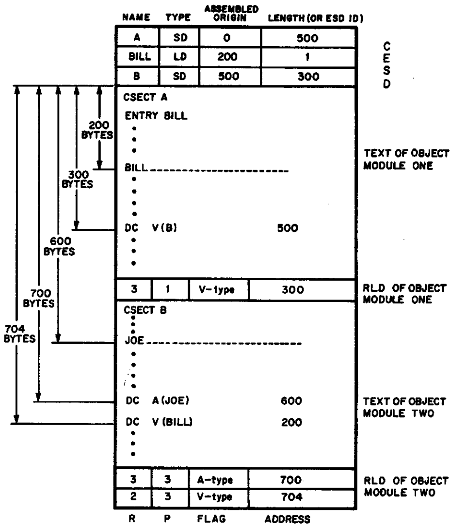
FIG. 9. Format of output Load Module.
